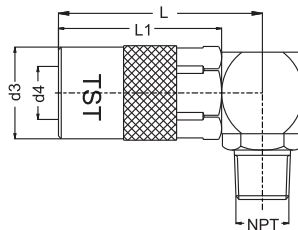
NPT Thread socket 45° Kupplung mit 90° Aussengewinde NPT
