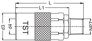
NPT Thread socket Kupplung mit Aussengewinde NPT
