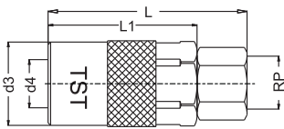
Cylindrical Thread socket Kupplung mit Innengewinde zylindrisch BSP
