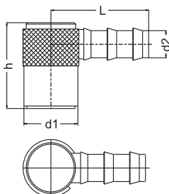
Flexible Diverting connector / Umlenkupplung mit Schnellsteck- Schlauchtülle
