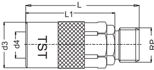
Cylindrical Thread socket Kupplung mit Aussengewinde zylindrisch BSP
