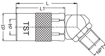
NPT Thread socket 45° Kupplung mit 45° Aussengewinde NPT
