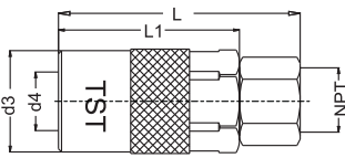
NPT Thread socket Kupplung mit Innengewinde NPT
