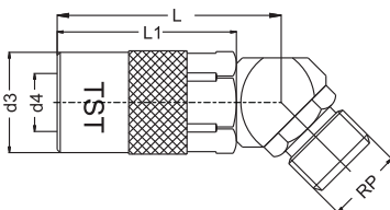
Cylindrical Thread socket 45° Kupplung mit 45° Aussengewinde zylindrisch BSP
